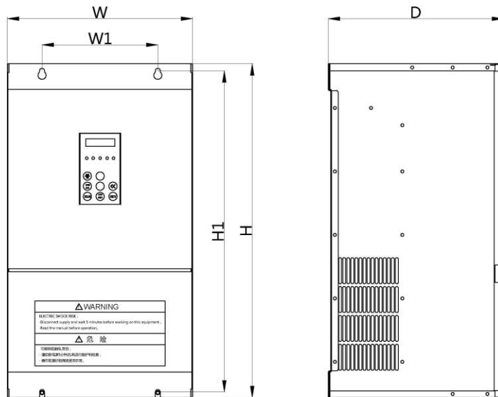
CV30 系列通用变频器外形尺寸和安装尺寸一览表
